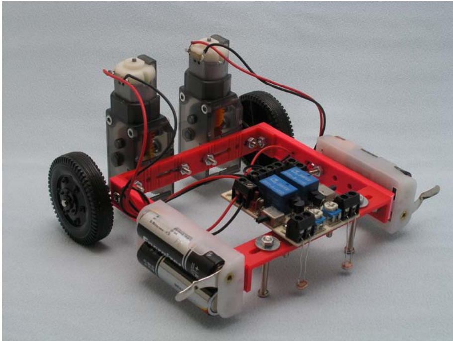
XBNC-001 黑線追蹤車(參考) (可另配 NC-002 第二代黑線追蹤器)
