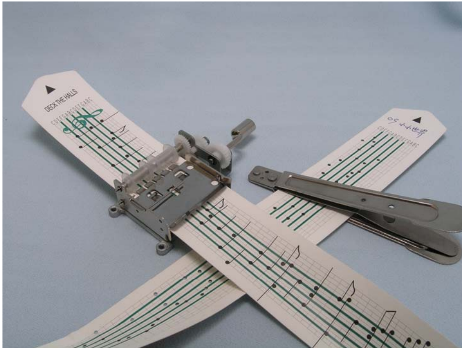
自編樂譜音樂機芯(附打孔器及紙帶 ZD15-01-1) HK$45.00/套 **另可配紙帶，每條 HK$2.00
