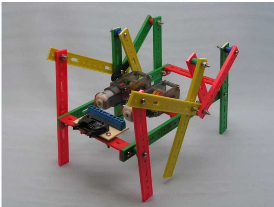
XB-602 膠製六足步行器(參考)
