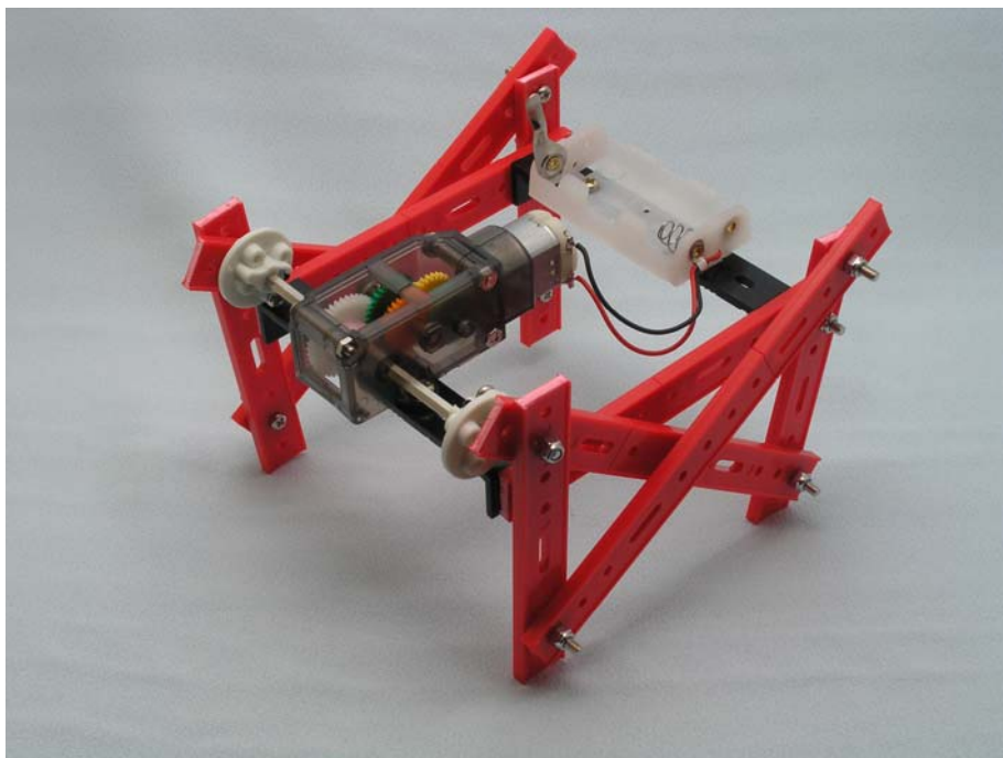
XB-402 膠製四足步行器(參考)
