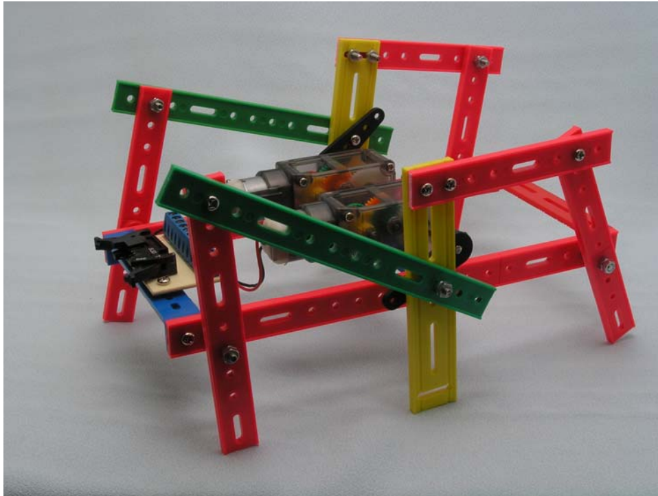
XB-601 膠製六足步行器(參考)
